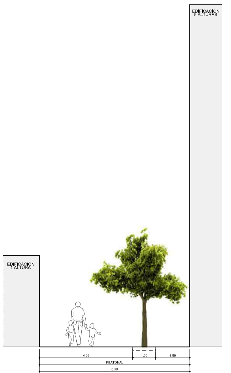
SECCIÓN E-E' (Calle Santiago)
