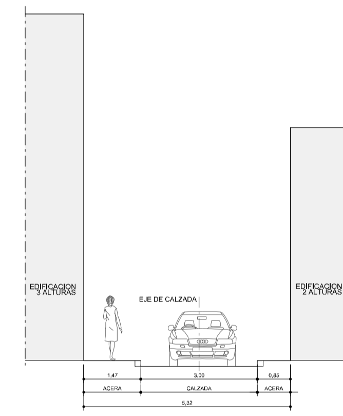
SECCIÓN K-K'
