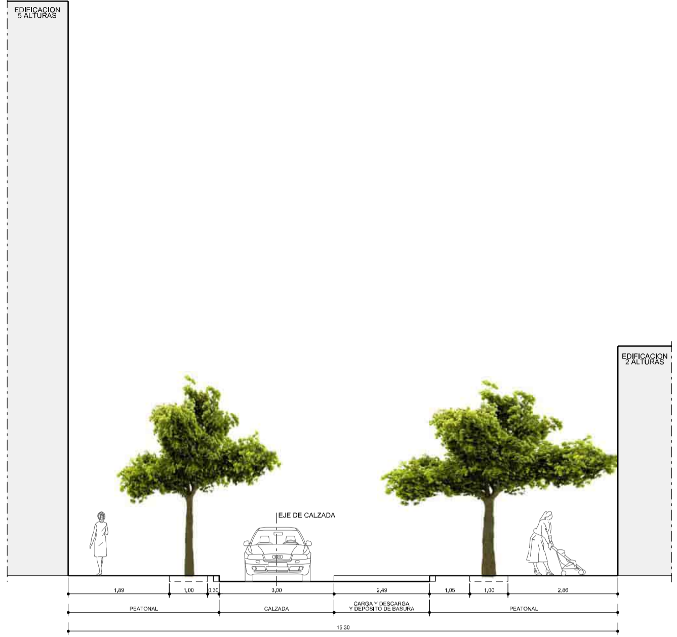
SECCIÓN A-A' (Calle La Rosa)
