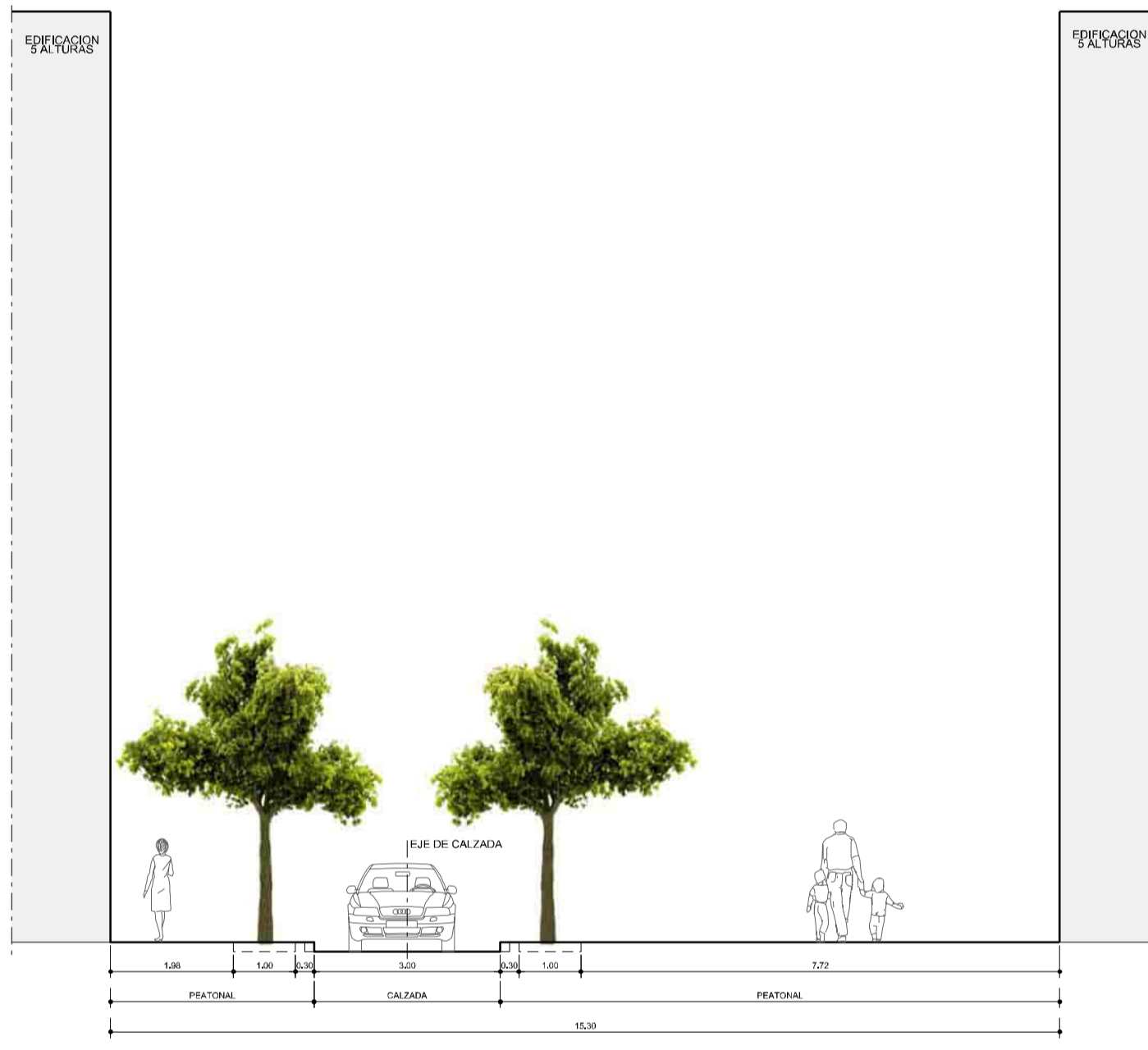
SECCIÓN C-C' (Calle La Rosa)
