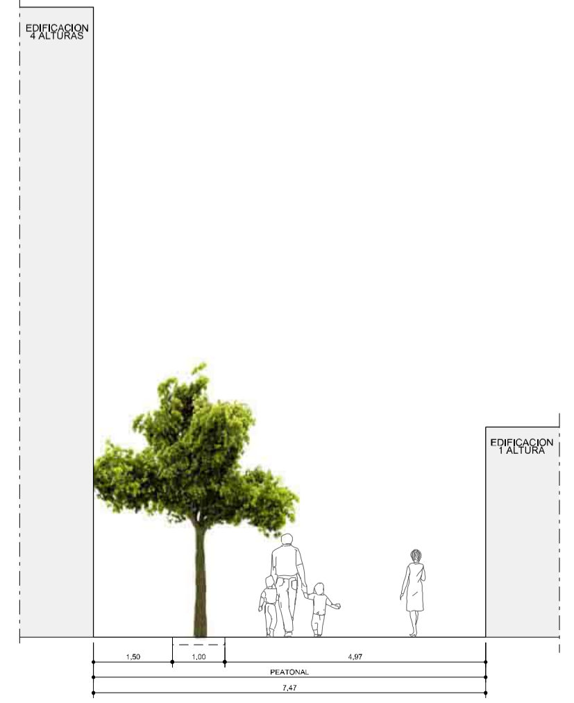
SECCIÓN F-F' (Calle San Miguel)
