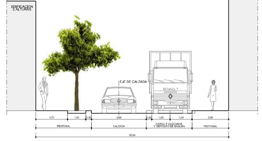
SECCIÓN B-B' (Calle La Rosa)
