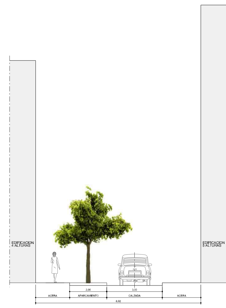
SECCIÓN H-H'
