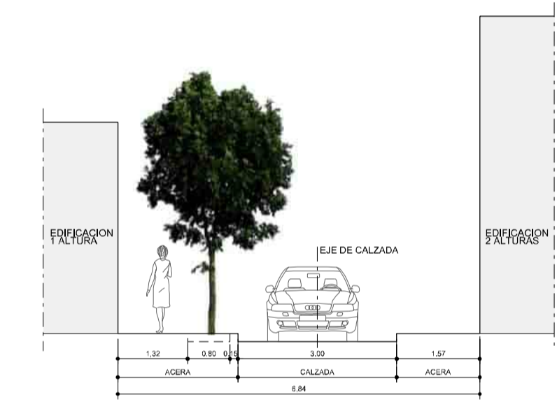
SECCIÓN J-J'
